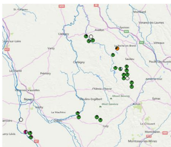
Carte 3 : Répartition géographique des groupes génétiques distincts mis en évidence en Bourgogne (en vert : le Limousin, en orange : la Bretagne et en violet : le massif central). Les diagrammes représentent pour chaque individu les probabilités d'appartenance à chacun des six groupes génétiques définis. Source : Lise-Marie PIGNEUR
